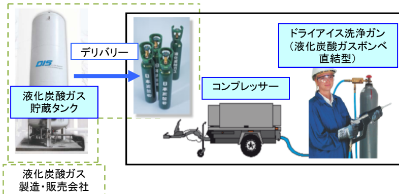
液化炭酸ガスポンベ直結型ドライアイスブラスト洗浄機
