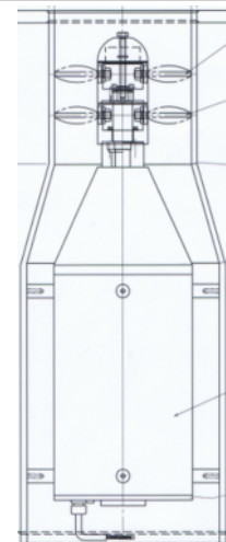
水力発電機 (断面図)
