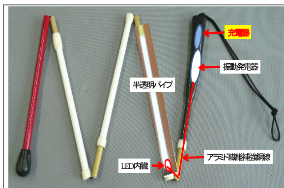
振動発電により点灯するLED付き白杖
