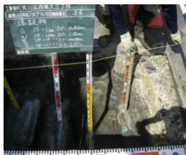
都市部の地下埋設状況
