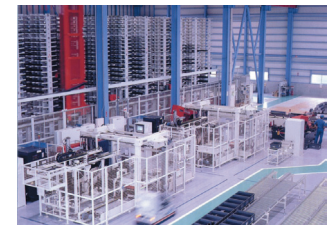
24 時間無人自動切断ライン
