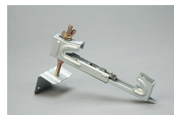
ワンタッチ固定式天井吊金物
