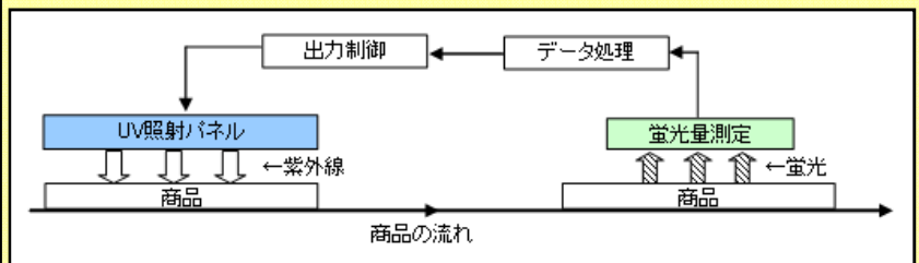
装置と加工品の流れ
