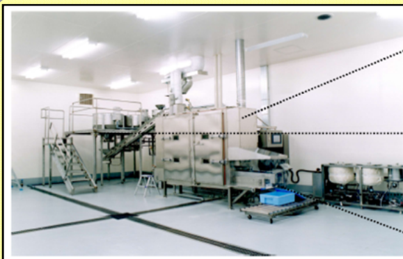
RM全自動連続蒸気炊飯機
