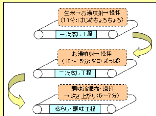
RM全自動連続蒸気炊飯機の構造と方式
