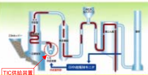
燃焼室付近に吹き込む場合の概念図
