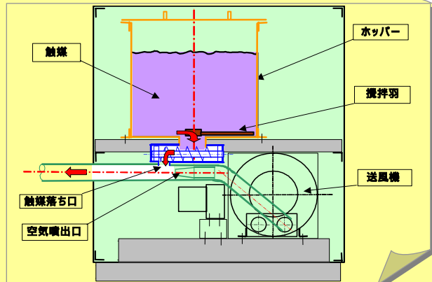
供給機要部の構造概念図
