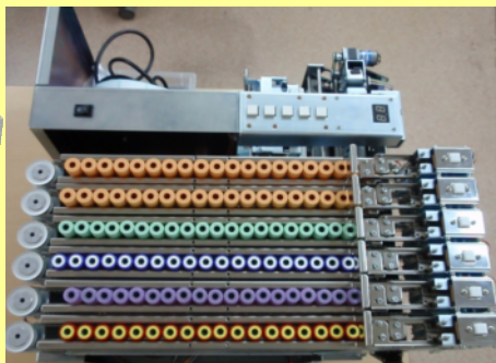
採血管の搬送と収容部分
