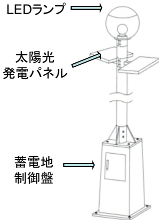
LED光リユース街路灯の構造
