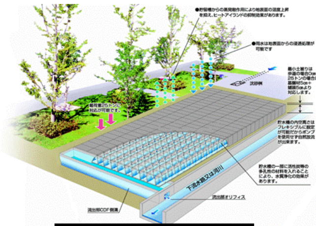
雨水地下貯留槽完成イメージ
