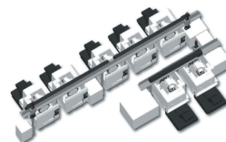
顧客ニーズに合わせてカスタマイズした切削加工自動化ライン
